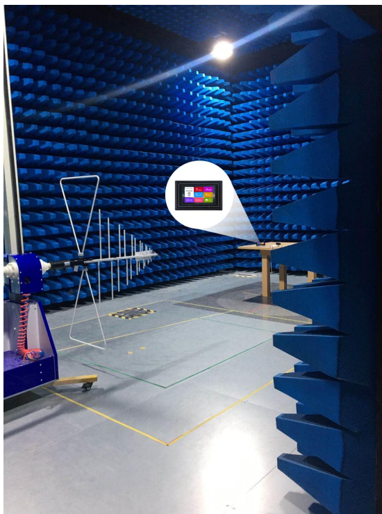
图 6-5 辐射测试图
